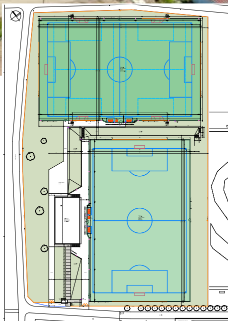
Le drainage en arête sur le terrain en gazon naturel
